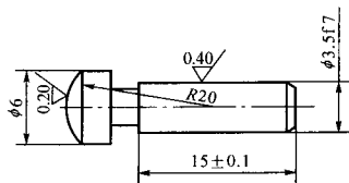
图 5 测力专用球面测头
