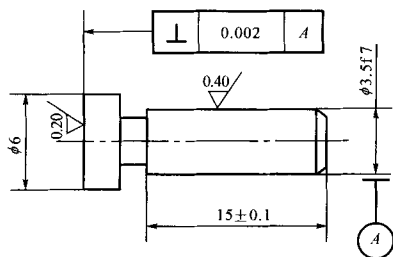
图 8 平面测头
