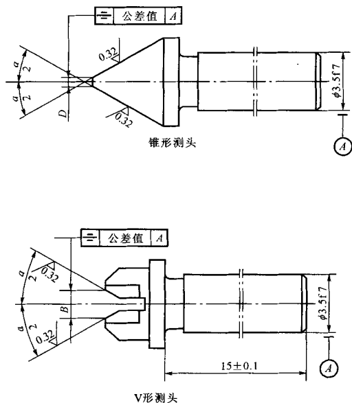
图 4 锥形测头及 V 形测头的尺寸
