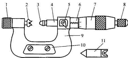
图1 标尺式螺纹千分尺结构
