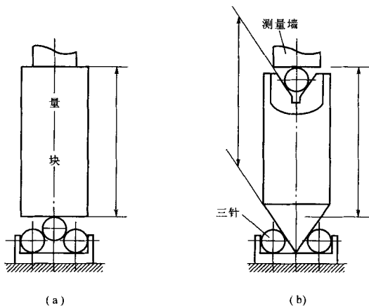
图 11 校对用量杆工作尺寸检定方法
