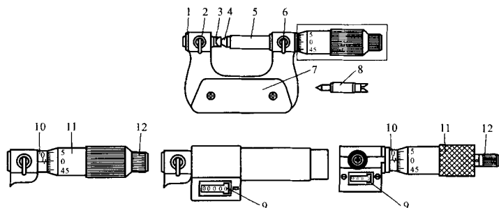
图2 数显式螺纹千分尺结构
