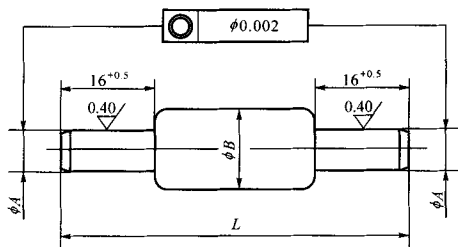
图 7 专用量规
